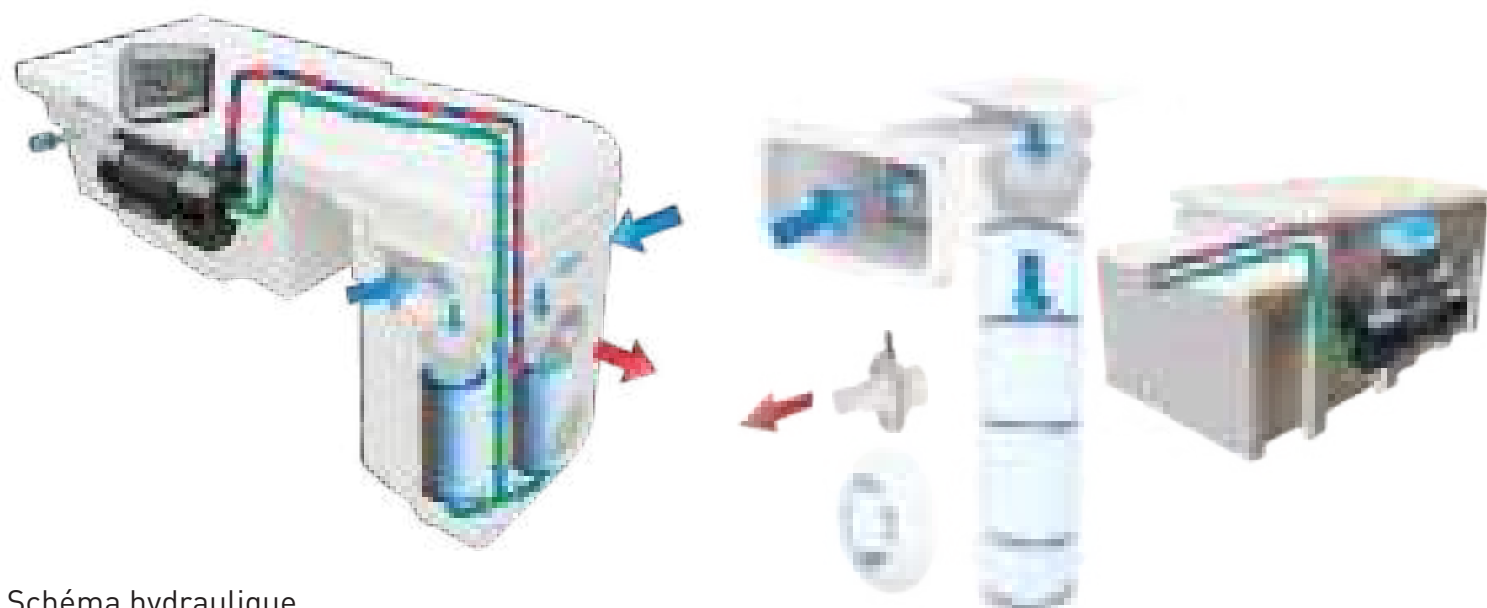
Schéma hydraulique du bloc filtrant (standard hors options)
